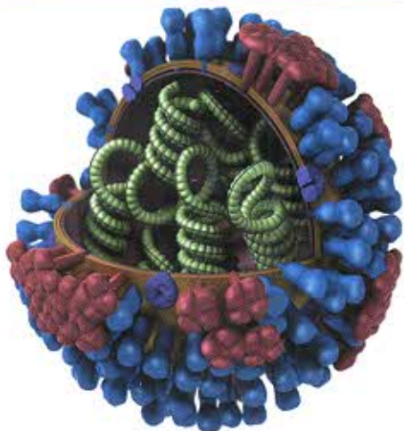
Hemagglutinin
